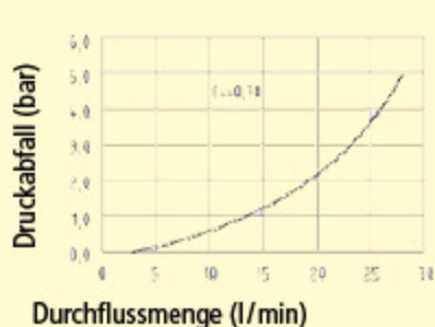
Durchflussdiagramm WASSER* Kuplungssystem ESER | ESEG DN 7.2 beidseitig absperrend
