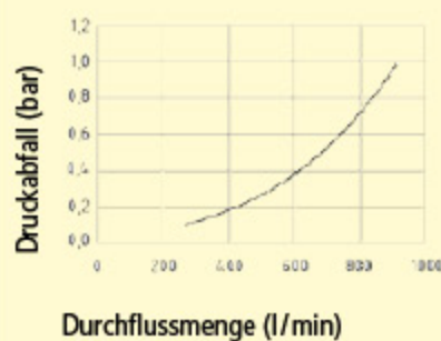
Durchflussdiagramm LUFT* Kuplungssystem ESER | ESEG DN 7.2 beidseitig absperrend
