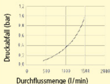
Durchflussdiagramm LUFT* Kuplungssystem ESER | ESEG DN 7.2 einseitig absperrend
