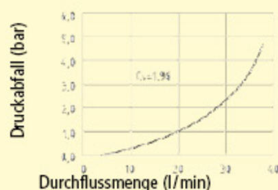
Durchflussdiagramm WASSER* Kuplungssystem ESER | ESEG DN 7.2 einseitig absperrend
